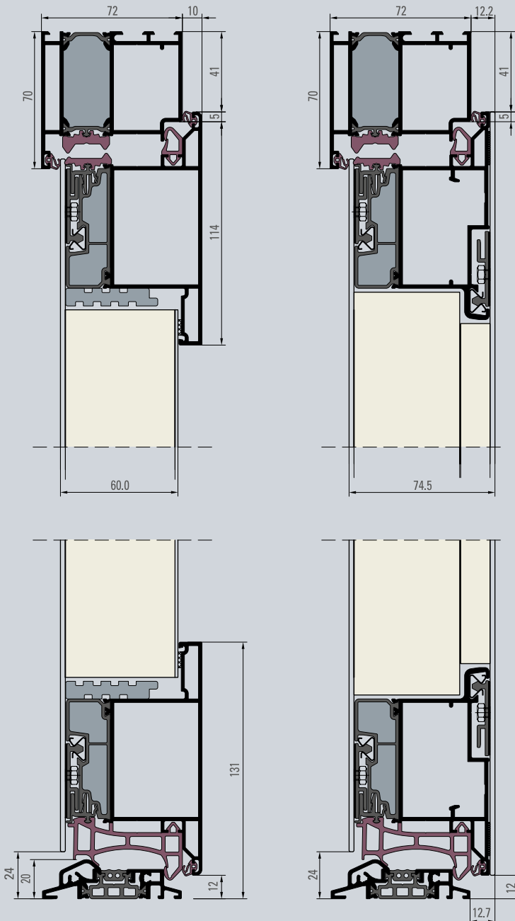
SMART AF (AUSSEN FLÜGELÜBERDECKEND) U_D AB 0,97 W/M 2 -K
