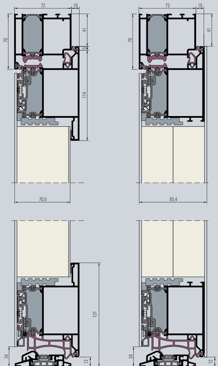
OBJEKT 3D AF (AUSSEN FLÜGELÜBERDECKEND) U_D AB 0,94 W/M 2 ·K
